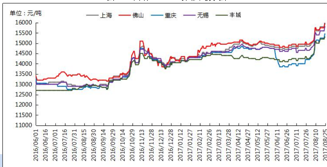
图3 国标ADC12价格走势
