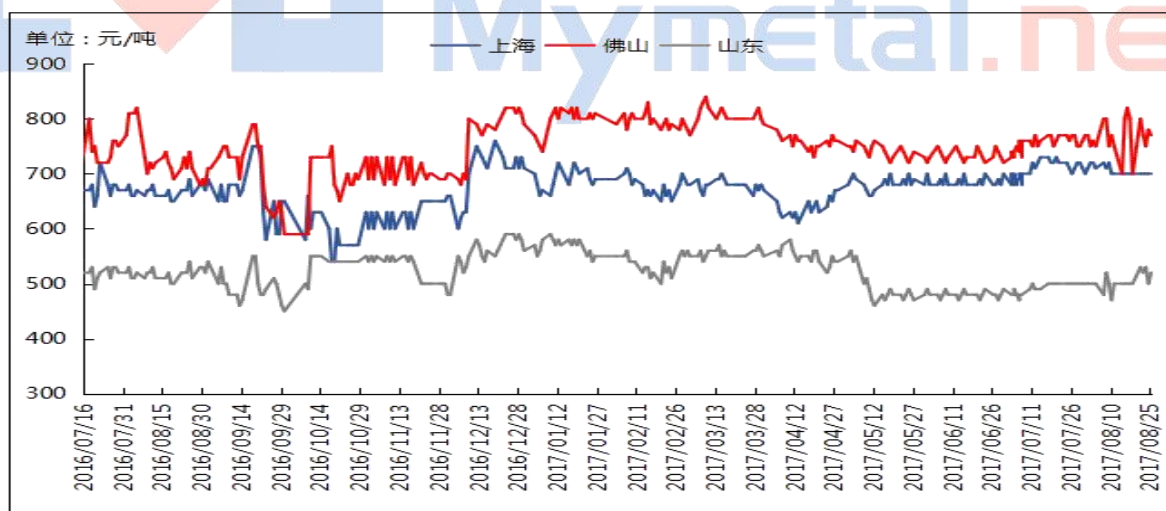
图5 全国主流地区 A356.2 铝合金锭加工费走势图 规格：国标
