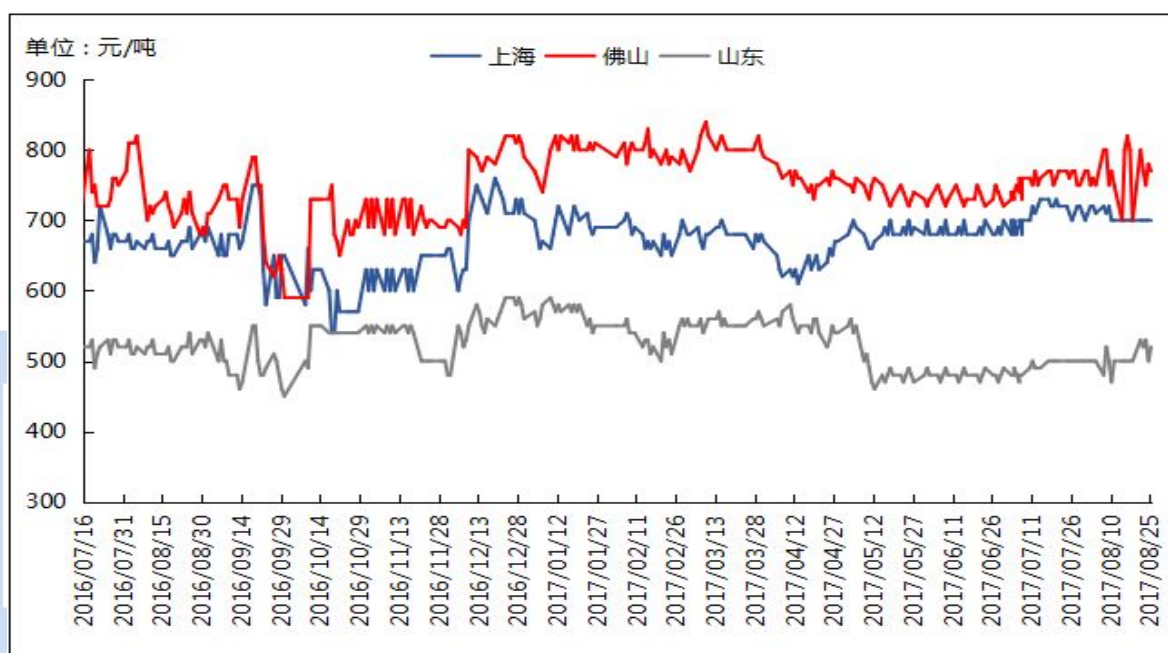
图7、全国主流地区 A356.2铝合金锭加工费走势图 规格：国标
