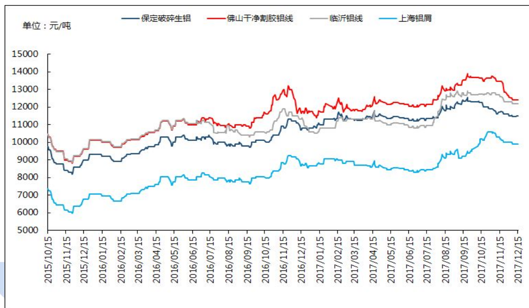
图5、 全国主流地区废铝价格走势图
