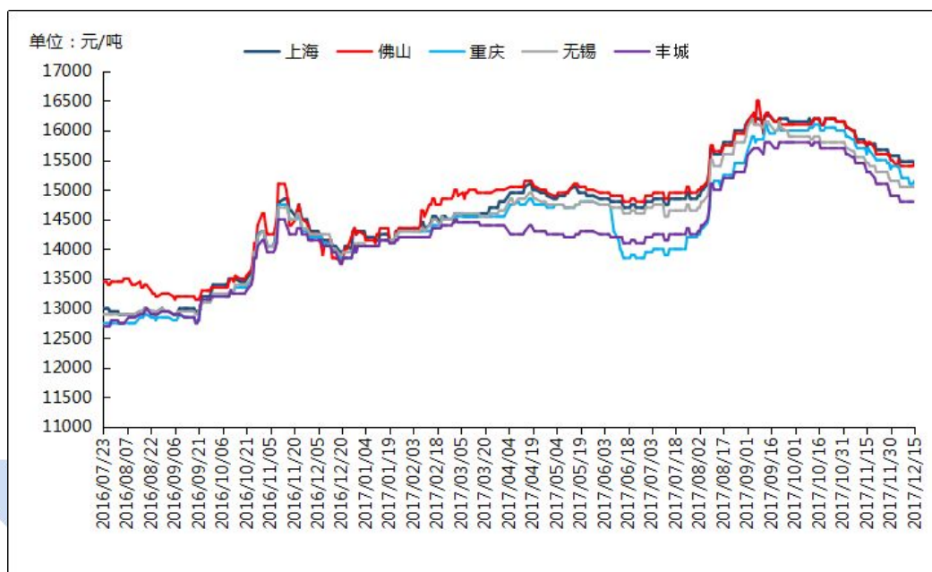
图6、全国主流地区国标 ADC12价格走势
