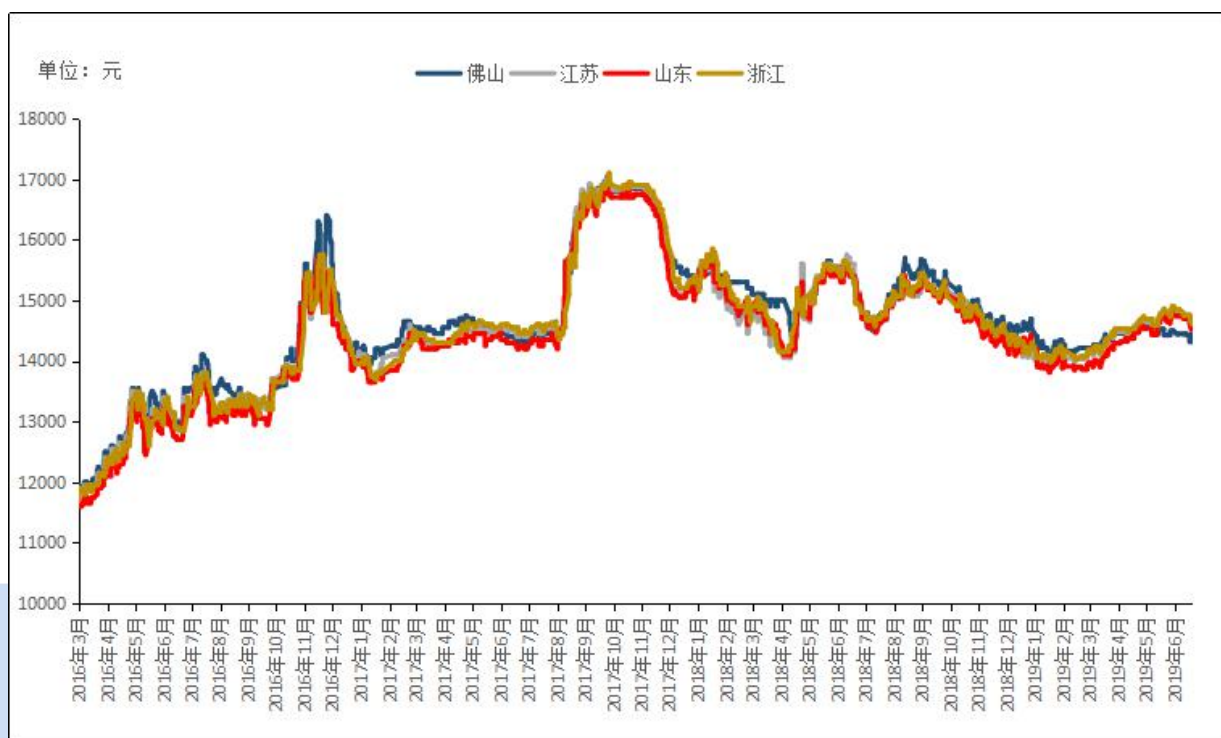
图3 全国主流地区 A356.2铝合金锭价格走势 规格：国标
