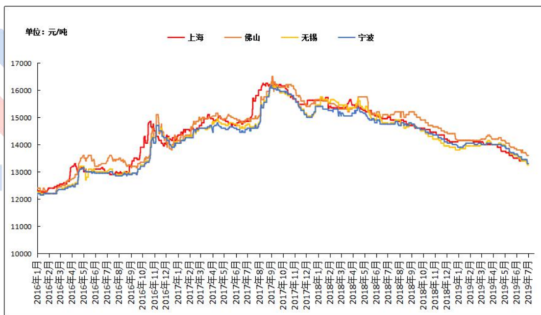
图2 全国主流地区国标 ADC12价格
