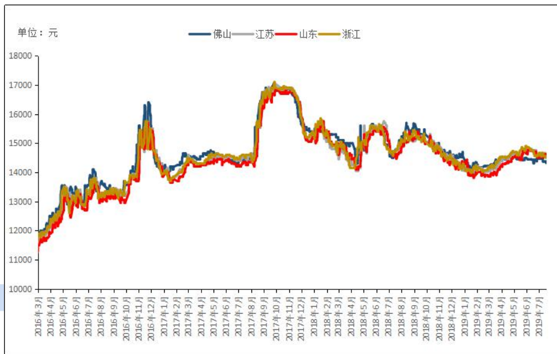
图3 全国主流地区 A356.2 铝合金锭价格走势 规格：国标
